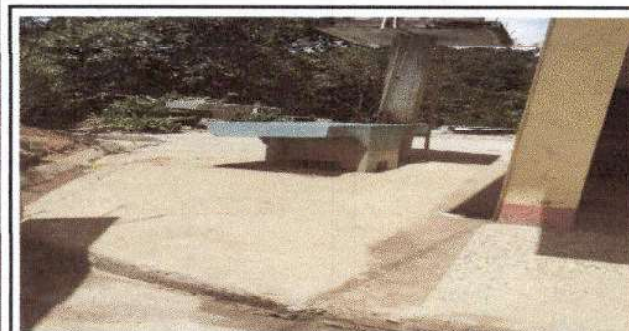
Foto 3: Reparación de planchas de concreto de patio.
